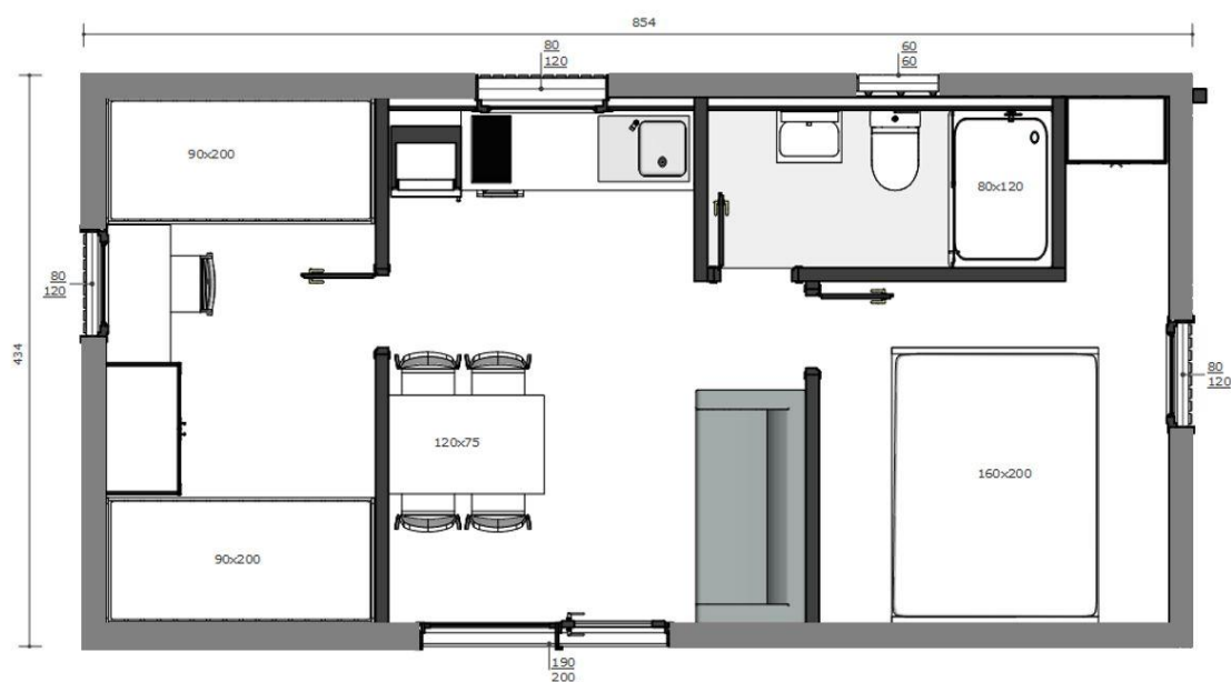
Tlocrt mobilne kuće Leona 36
